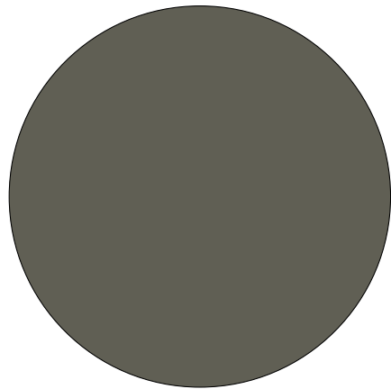
Callisto
